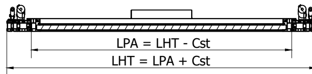
B-B ( 1:12 )
