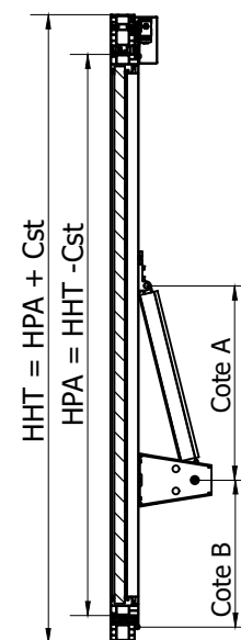
A-A ( 1:12 )
